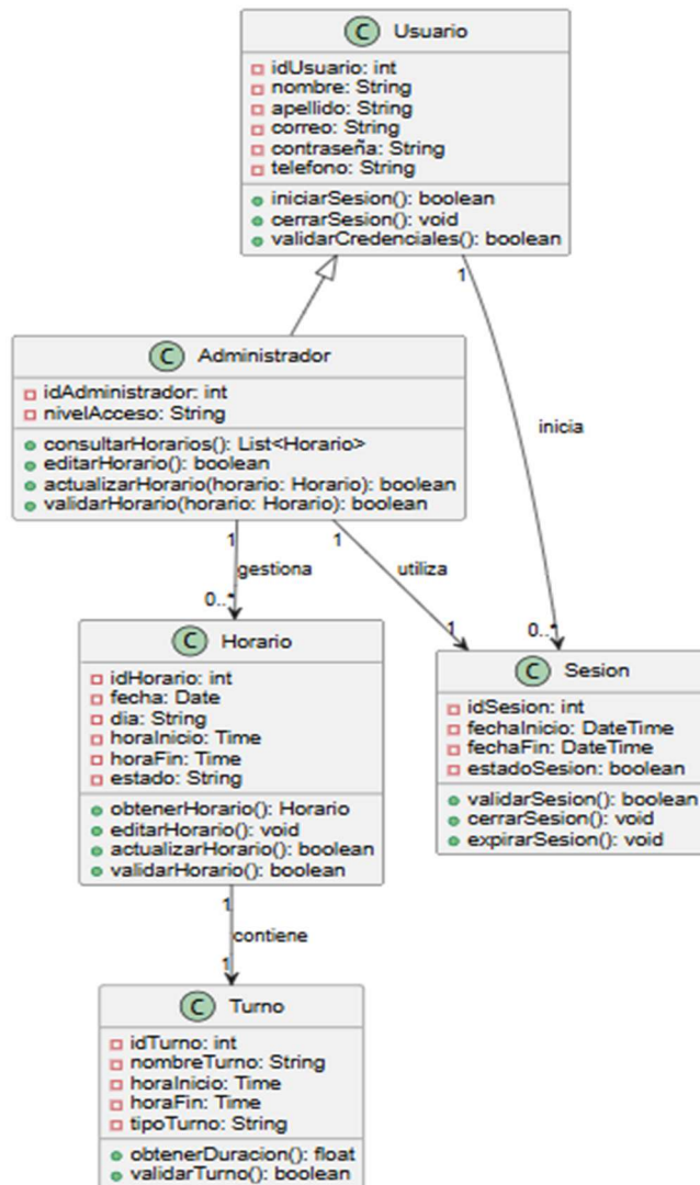
Diagrama de Clases - RF11 Editar Horario
